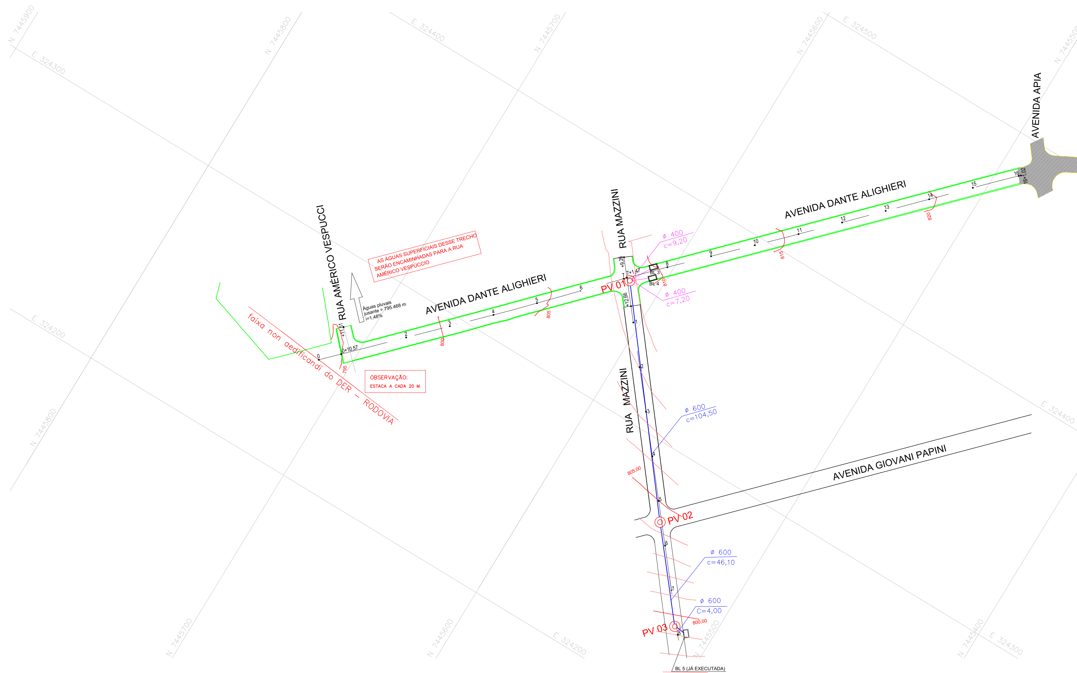
TRECHO 1 PROJETO DE DRENAGEM ESC. 1:1.000
